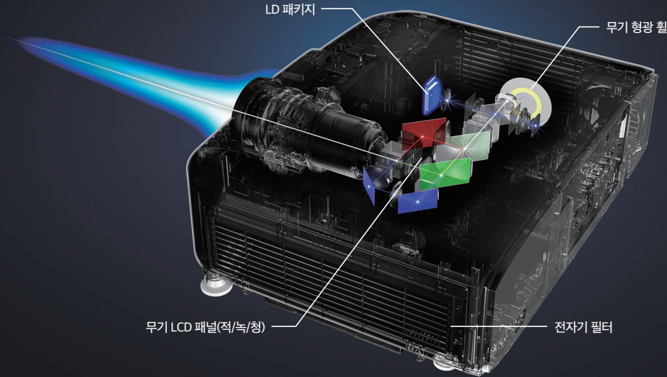
LD(레이저 다이오드) 패키지
